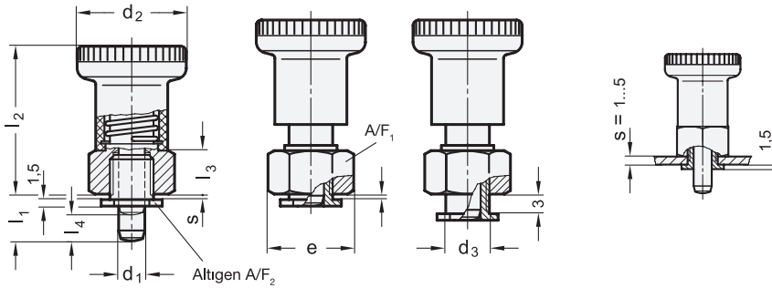
Geri çekilmiş piston pimi
